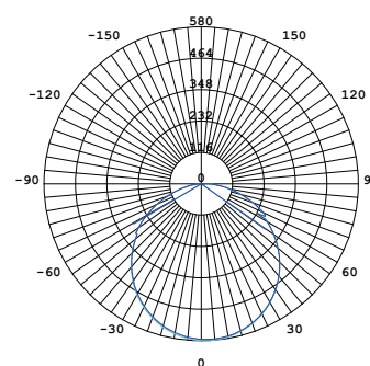
CURVA FOTOMETRICA
